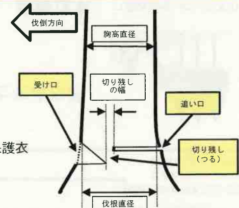
（図2）受け口、追い口等の関係図
