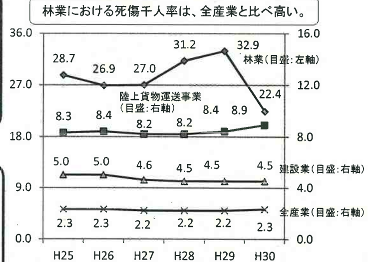
《図2》 林業における作業の種類別死亡者数(平成27-28年発生分79人の内訳)
